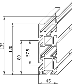
124 AL
