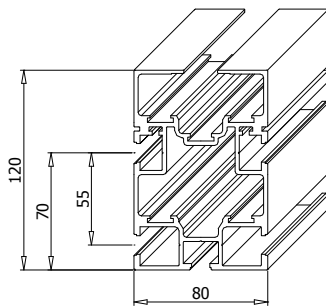
128 AL
