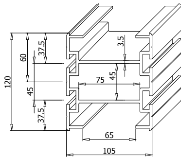
105 AL
