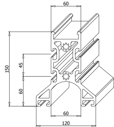
150 AL-K
