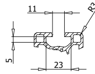
Nut Groove
