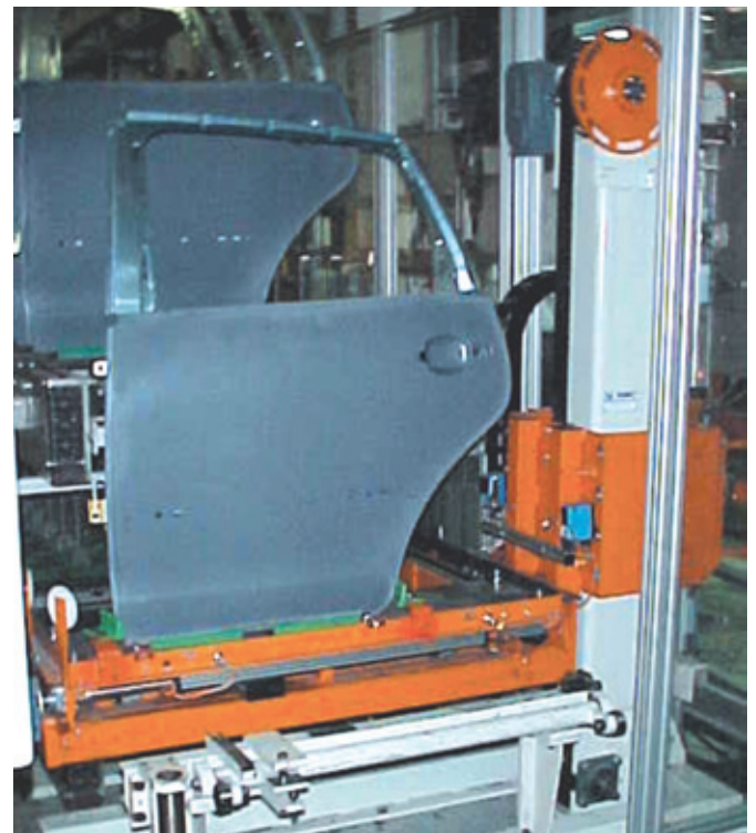
Zuführung der linken Hintertür Feeding of left rear door
