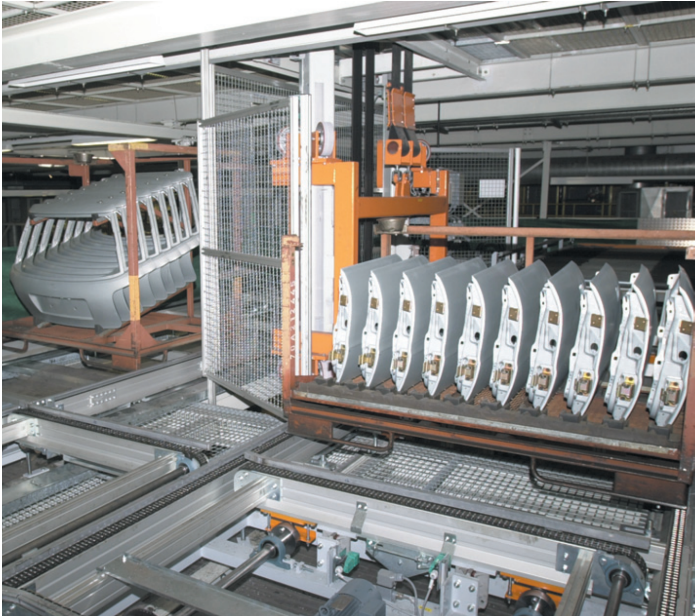
Heber und Kettenförderer für Transportgestelle Türen Lifters and chain conveyors for door-transporting frames
