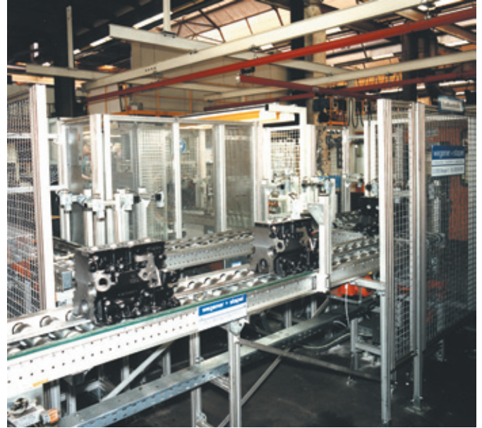
VW, Salzgitter: Fördereinrichtung für Motoren-Prüfeinrichtung VW, Salzgitter: Conveying system for motor test unit
