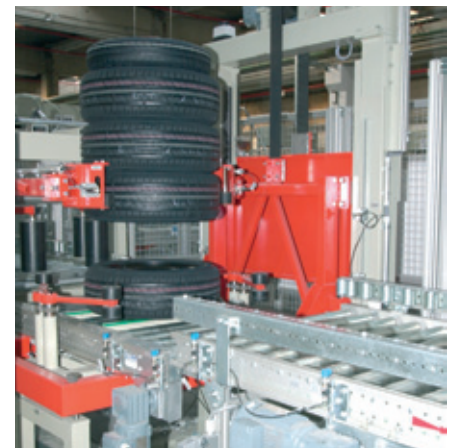
Räderstapler mit Ausrichteinheit Wheel stacker with alignment unit
